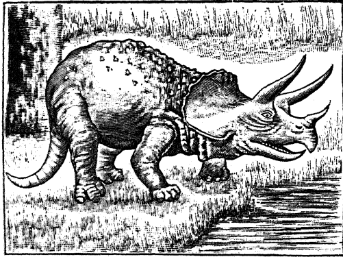
चित्र २४—प्राचीन गैंडा
